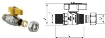
ART. 1220 M x OLIVE EN 331 DVGW
