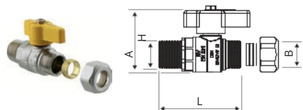
ART. 1220 M x OGIVA EN 331 DVGW
