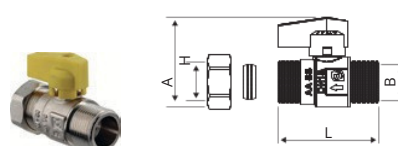
ART. 1220/B M x F
