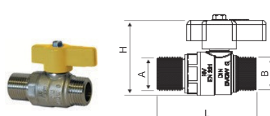
ART. 1222/AD M x M
