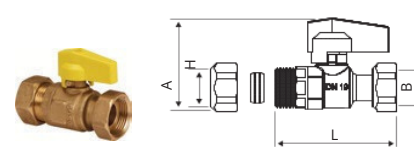
ART. 1225 OGIVA x F
