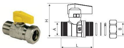
ART. 1223 M x OGIVA
