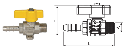
ART. 1220/PF M EN 331 DVGW
